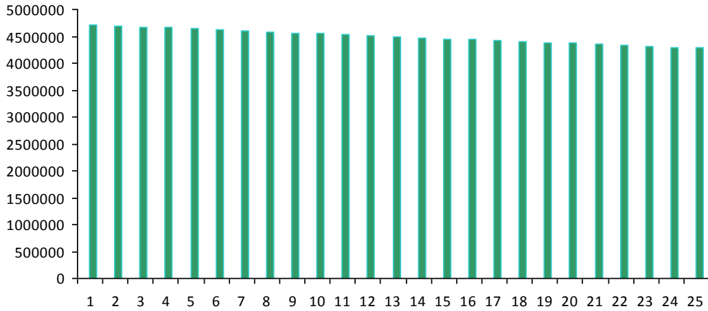
Şekil 6.3. 3 MW'lık PV Sisteminden Karapınar'da Üretilecek Yıllık Toplam Elektrik Enerjisi (kWh)
